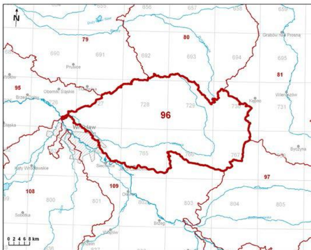
Ryc. 3. Zasięg JCWPd 96.
