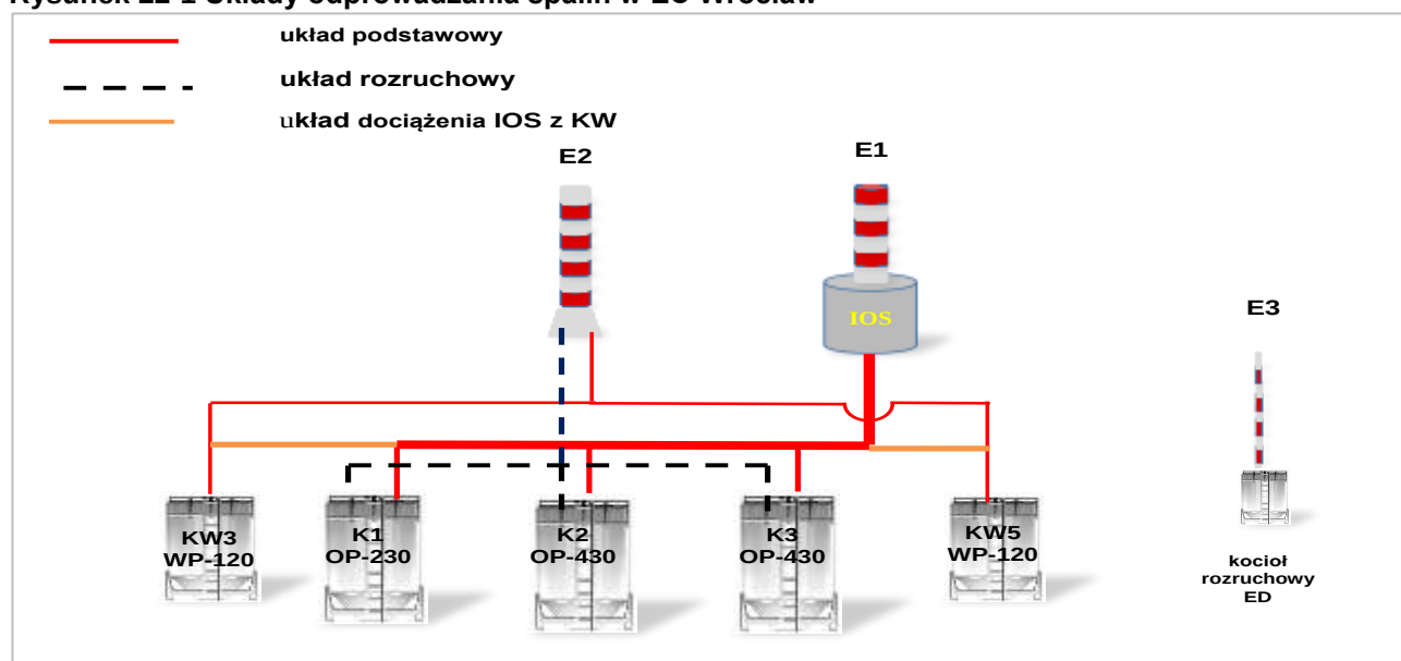
Rysunek 22-1 Układy odprowadzania spalin w EC Wrocław
