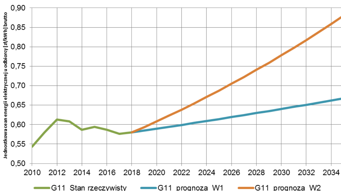
Wykres 11-16 Prognoza cen energii elektrycznej
