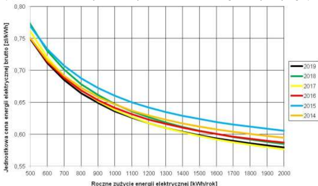
Wykres 11-2 Porównanie jednostkowych kosztów brutto energii elektrycznej w grupie G11
