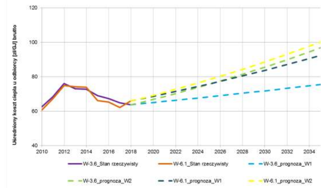
Wykres 11-12 Prognoza uśrednionych kosztów ciepła z gazu sieciowego
