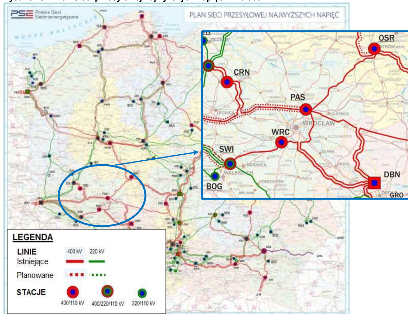
Rysunek 5-1 Plan sieci przesyłowej najwyższych napięć w Polsce
