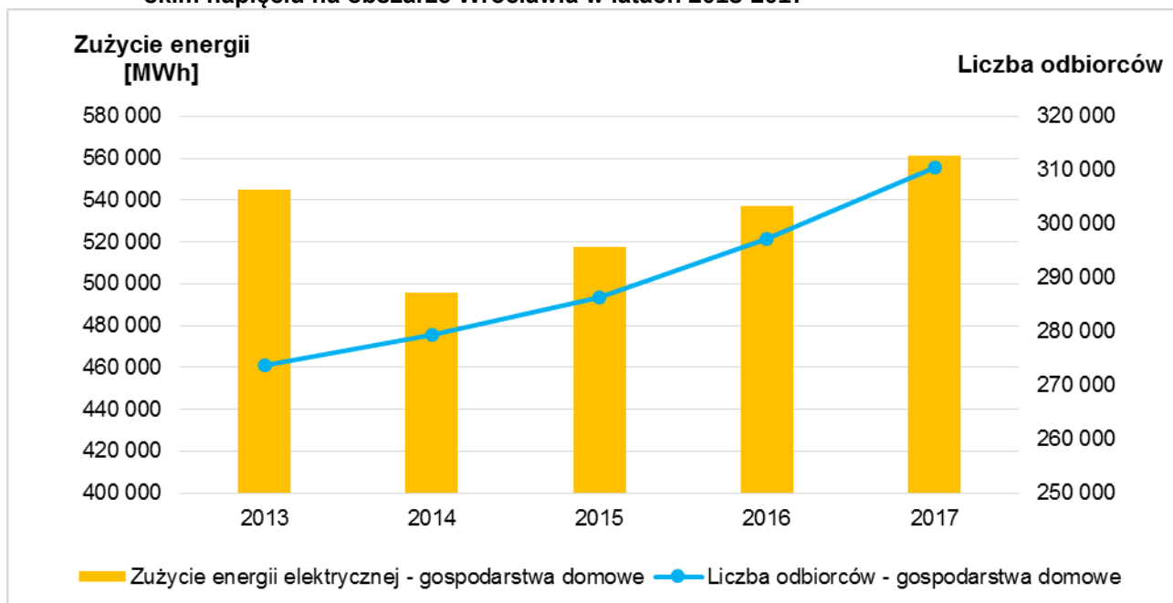
Wykres 5-3 Liczba odbiorców i zużycie energii elektrycznej w budownictwie mieszkaniowym na niskim napięciu na obszarze Wrocławia w latach 2013-2017
