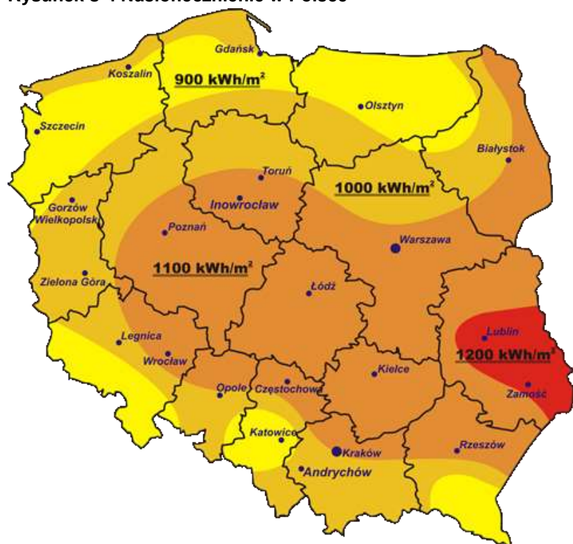
Rysunek 8-4 Nasłonecznienie w Polsce
