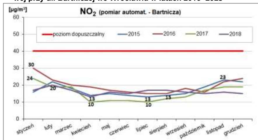
Wykres 21-11 Rozkład stężeń dwutlenku azotu mierzonych metodą automatyczną na stacji pomiarowej przy ul. Bartniczej we Wrocławiu w latach 2015÷2018
