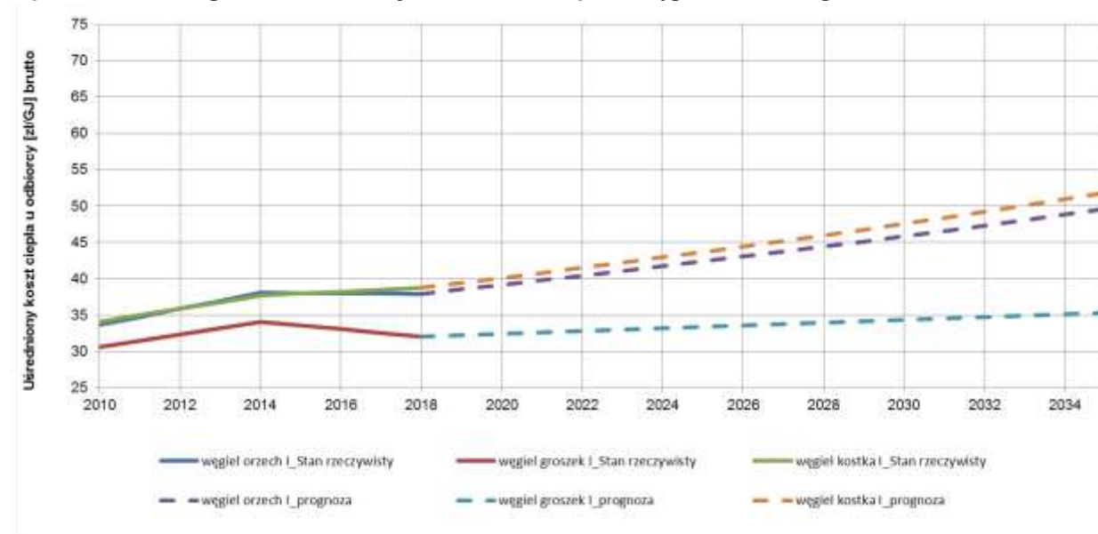
Wykres 11-14 Prognoza uśrednionych kosztów ciepła z węgla kamiennego
