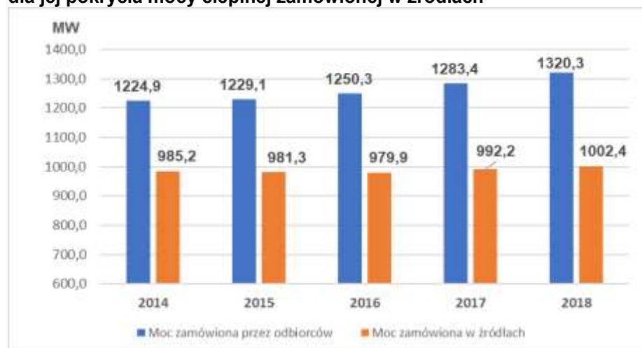
Wykres 4-4 Skala zmian mocy cieplnej zamówionej przez odbiorców z terenu Wrocławia i wymaganej dla jej pokrycia mocy cieplnej zamówionej w źródłach
