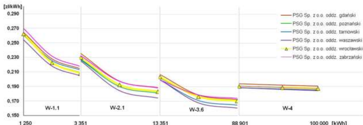
Wykres 11-6 Jednostkowa cena brutto [zł/kWh] zakupu gazu dla grup taryfowych W-1.1 do W-4
