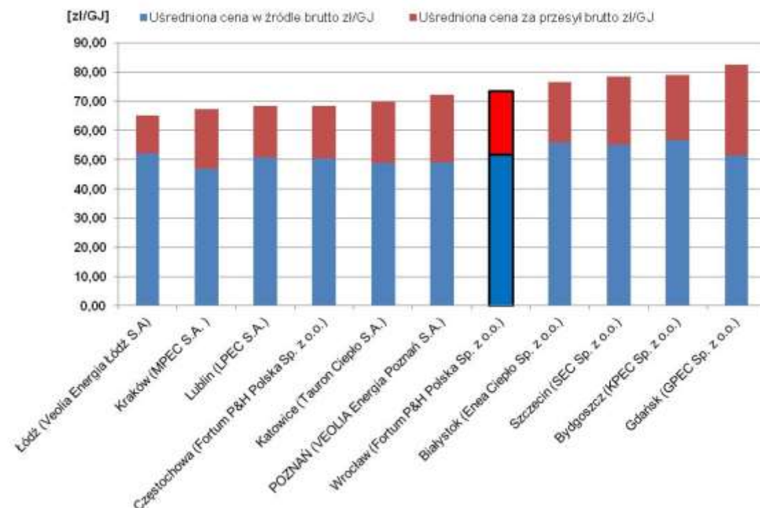
Wykres 11-1 Porównanie uśrednionych kosztów ciepła
