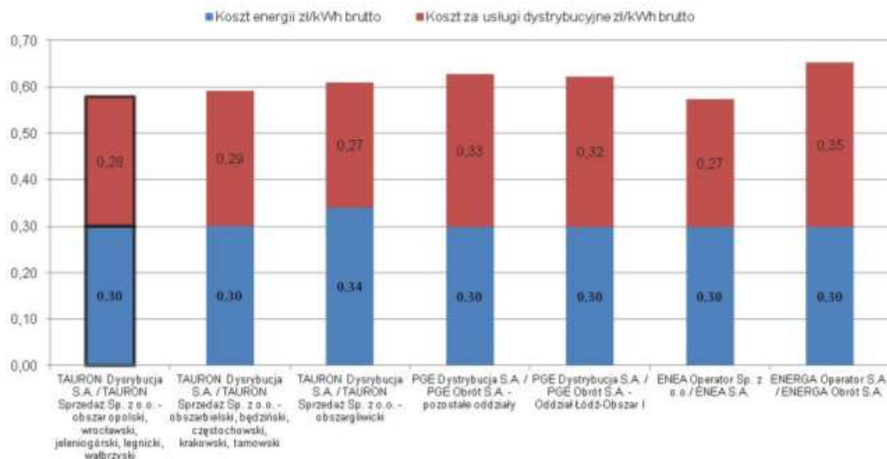
Wykres 11-5 Porównanie jednostkowych kosztów brutto energii elektrycznej w grupie G11 na tle innych przedsiębiorstw
