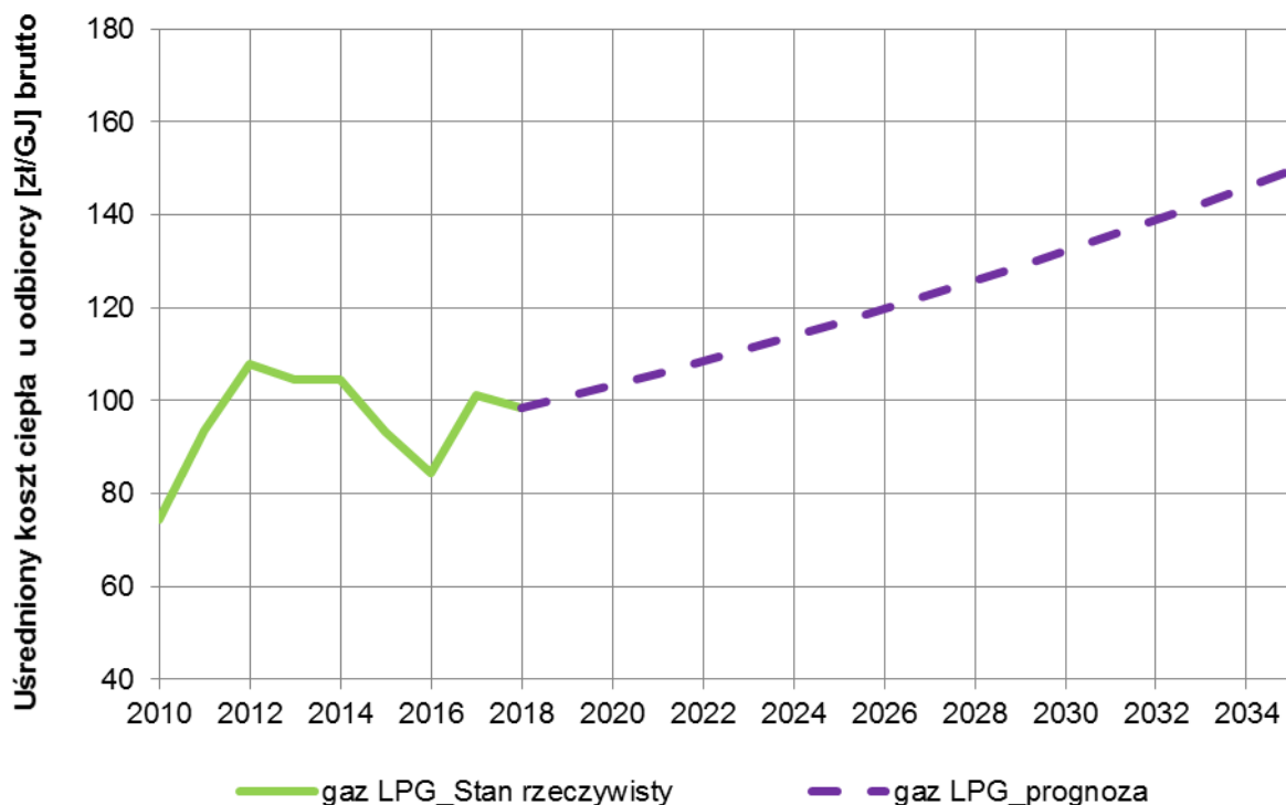
Wykres 11-13 Prognoza uśrednionych kosztów ciepła z gazu płynnego (LPG)
