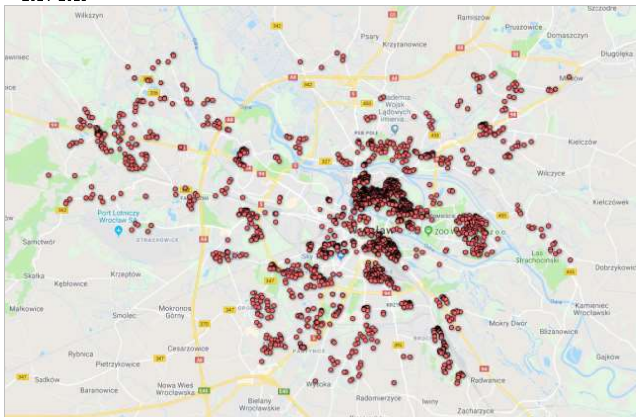
Rysunek 22-2 Mapa gęstości zlikwidowanych we Wrocławiu źródeł ciepła na paliwa stałe w latach 2014÷2018
