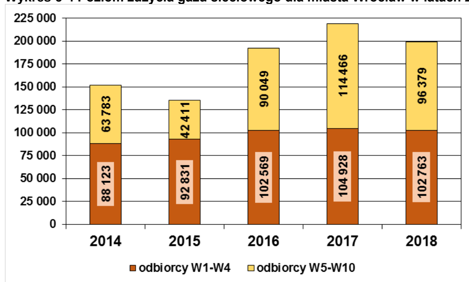
Wykres 6-4 Poziom zużycia gazu sieciowego dla miasta Wrocław w latach 2014-2018 [tys. m 3 ]
