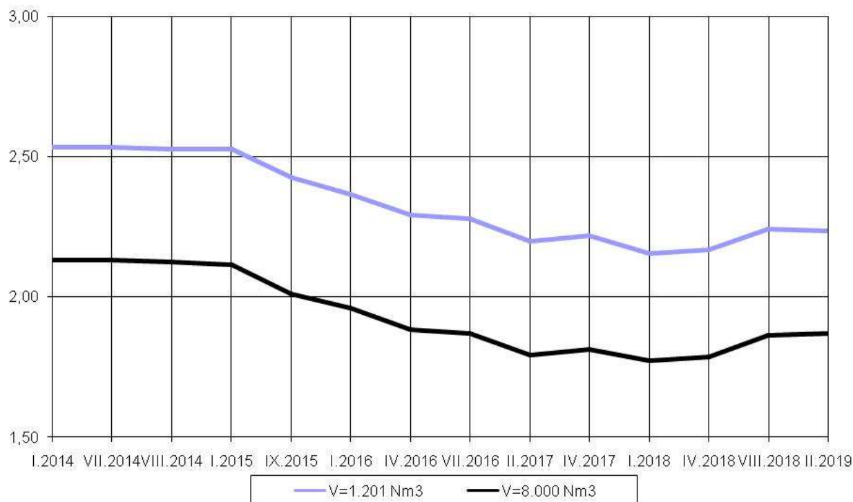
Wykres 11-10 Jednostkowy cena zakupu gazu w grupie taryfowej W-3.6 [zł/Nm 3 ]
