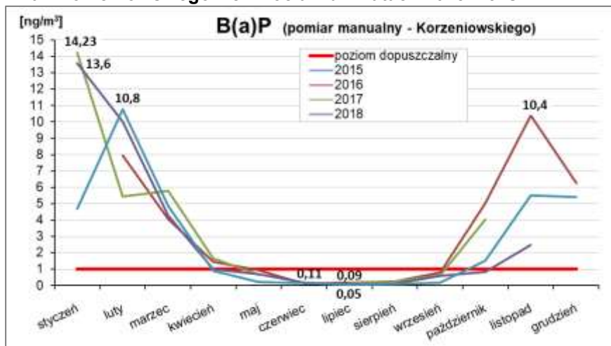
Wykres 21-7 Rozkład stężeń benzo(a)pirenu mierzonych metodą manualną na stacji pomiarowej przy ul. Korzeniowskiego we Wrocławiu w latach 2015÷2018
