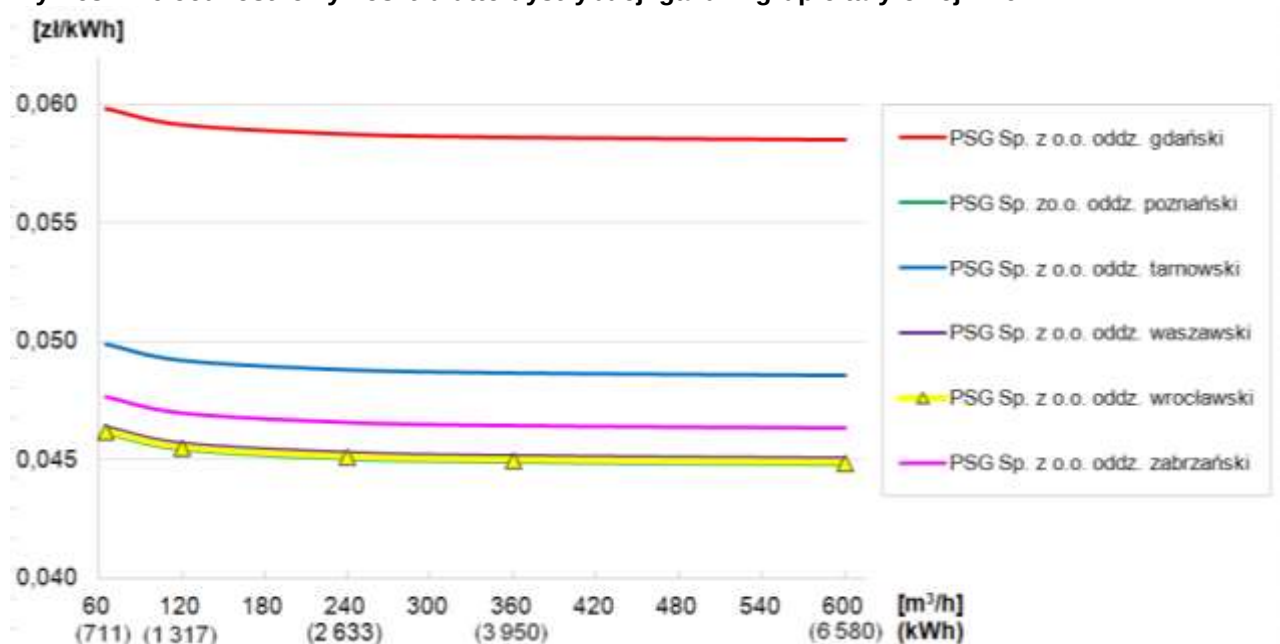
Wykres 11-9 Jednostkowy koszt brutto dystrybucji gazu w grupie taryfowej W-6A
