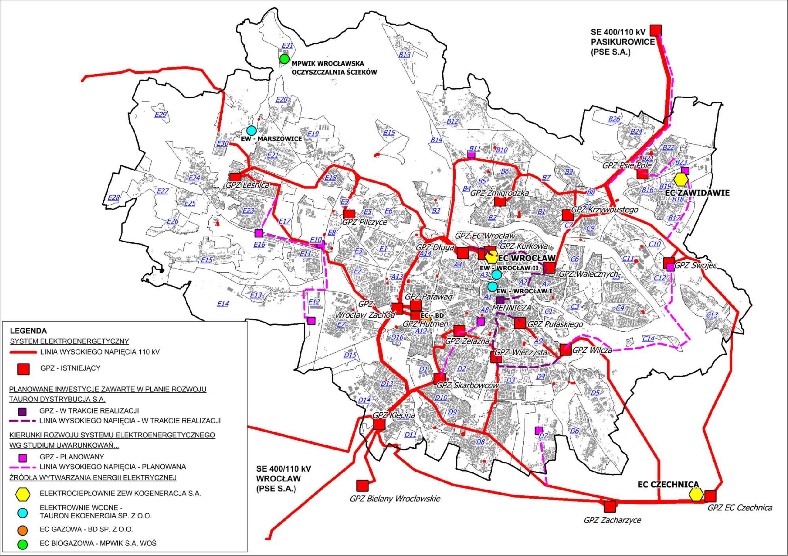
Mapa - System elektroenergetyczny
