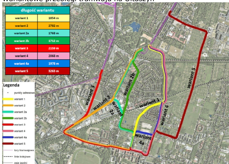
Wariantowe przebiegi tramwaju na Ołtaszyn
