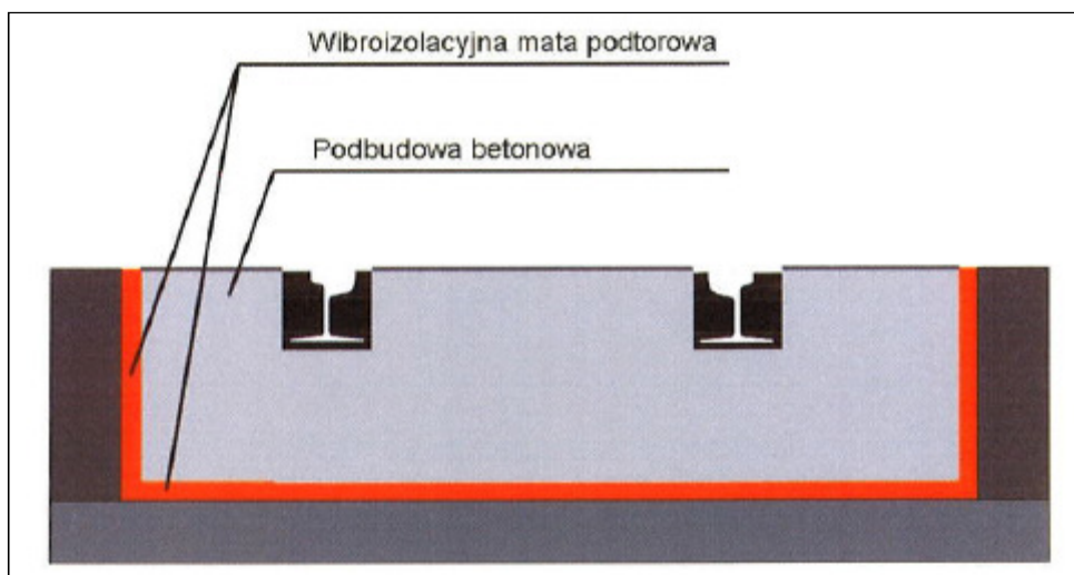
Rysunek 25. Przykład schematu zastosowania maty wibroizolacyjnej ( http://www.tines.pl ).
