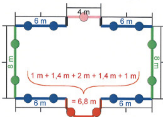
Rysunek 21. Sposób rozmieszczenia odbiorników na fasadach budynków mieszkalnych.
