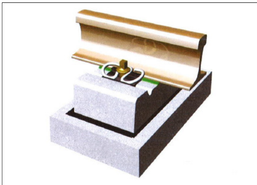
Rysunek 23. Przykładowy system podpór blokowych w otulinie ( http://www.tines.pl ).
