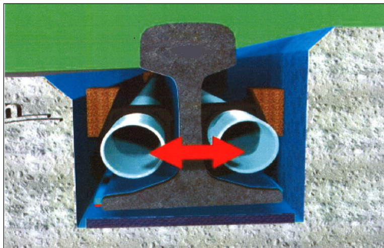
Rysunek 22. Przykład systemu szyny w otulinie ( http://www.tines.pl ).
