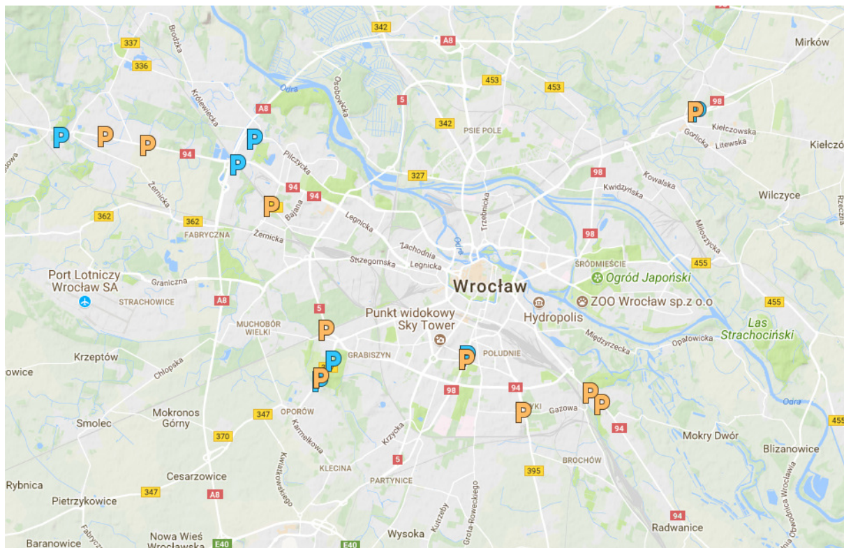
Rysunek 29. Lokalizacja wielkopowierzchniowych parkingów dla systemu P&R (kolor niebieski – istniejące parkingi, kolor zielony – planowane parkingi).
