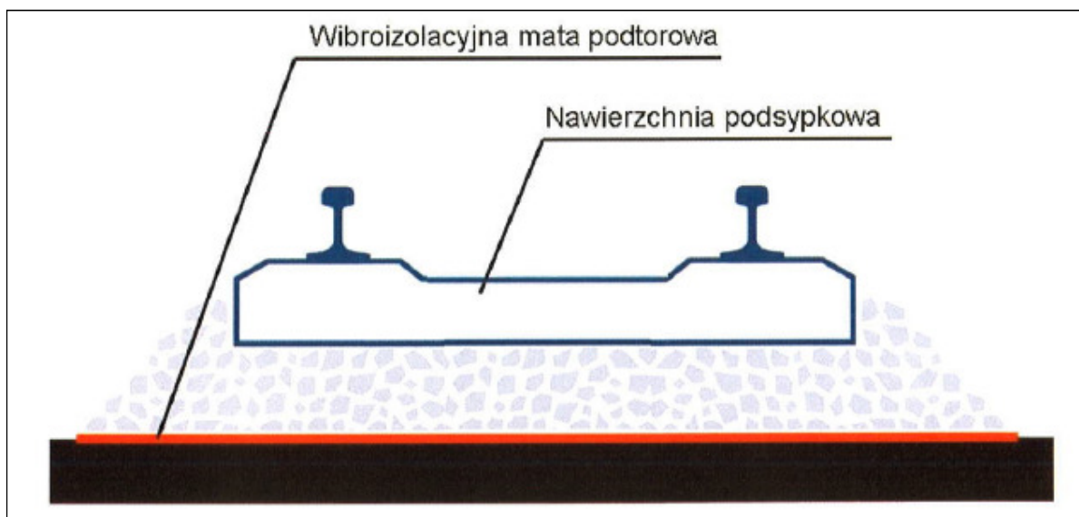
Rysunek 24. Schemat zastosowania maty wibroizolacyjnej ( http://www.tines.pl ).
