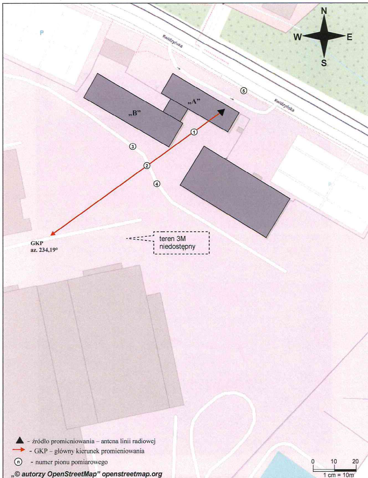
Rys. 1. Usytuowanie punktów i pionów pomiarowych w otoczeniu instalacji radiokomunikacyjnej Stacja Netia WROCD091-WROCM00906 Wrocław, ul. Kwidzyńska 6
