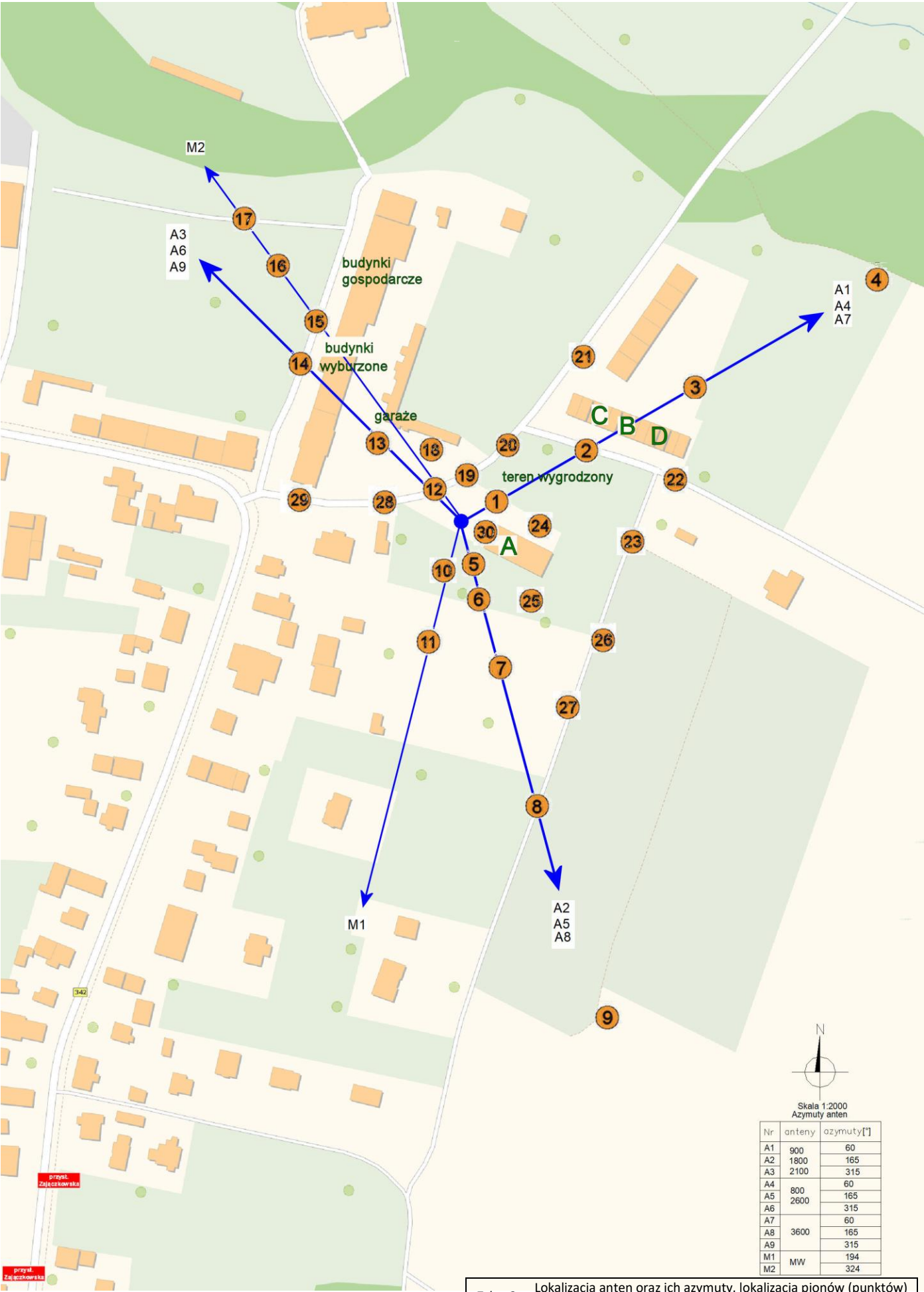
Załącznik nr 2: Lokalizacja anten oraz ich azymuty, lokalizacja pionów (punktów) pomiarowych wokół instalacji radiokomunikacyjnej. -punkt (pion) ● pomiarowy.
