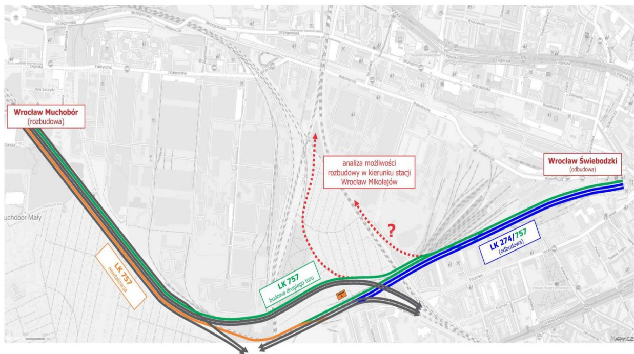
Rysunek 22. Planowany zakres rozbudowy linii kolejowej na terenie Wrocławia
