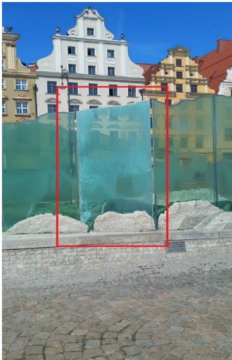
Fotografia 84. Fontanna na placu Gołębim przed naprawą
