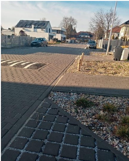
Fotografia 1. Ulica Przemysłowska po realizacji inwestycji
