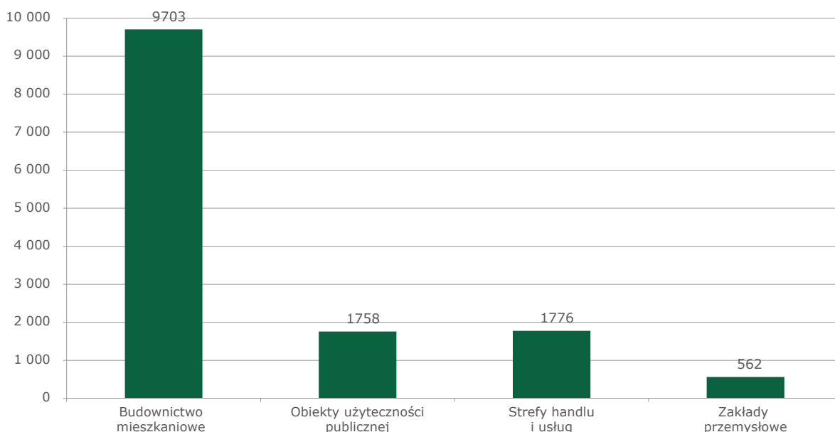
Wykres 55. Założenia do Planu zaopatrzenia w ciepło, energię elektryczną i paliwa gazowe dla obszaru Gminy Wrocław na lata 2020–2035; zapotrzebowanie na ciepło według grup odbiorców – roczne zużycie ciepła wyrażone jako roczne zapotrzebowanie u odbiorców (TJ)
