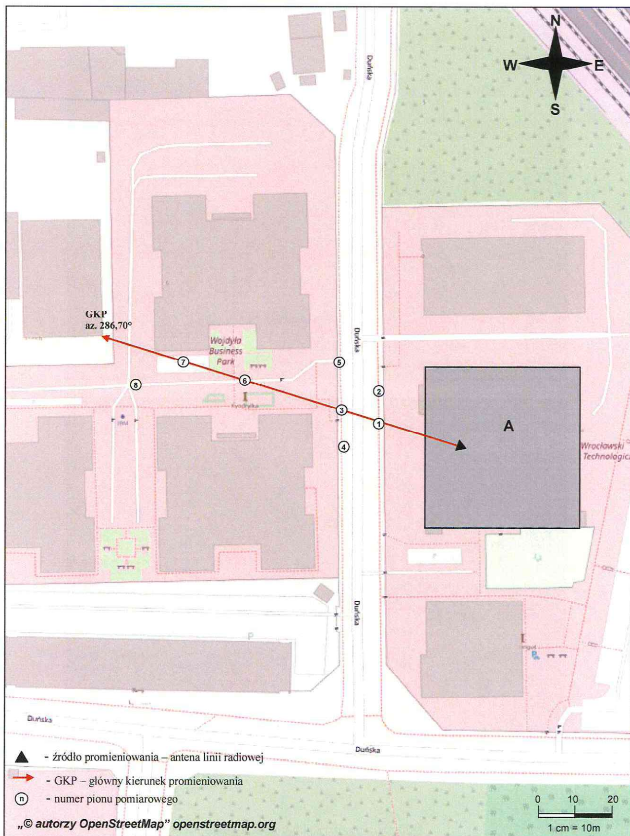
Rys. 1. Usytuowanie punktów i pionów pomiarowych w otoczeniu instalacji radiokomunikacyjnej Stacja Netia WROWD928-WROCM00900 Wrocław, ul. Duńska 9
