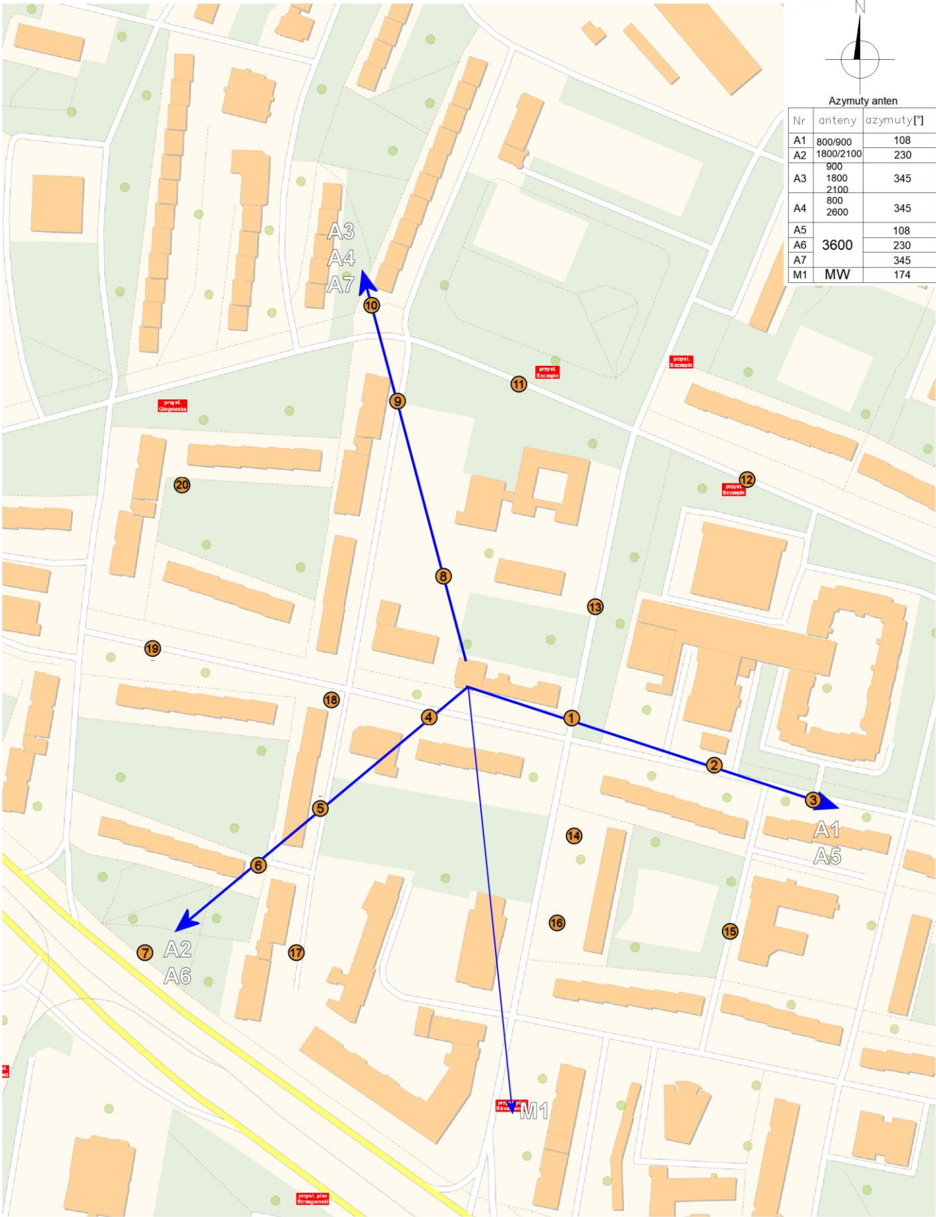
Załącznik nr 2: Lokalizacja anten oraz ich azymuty, lokalizacja pionów (punktów pomiarowych) wokół instalacji radiokomunikacyjnej. -punkt (pion) ● pomiarowy.
