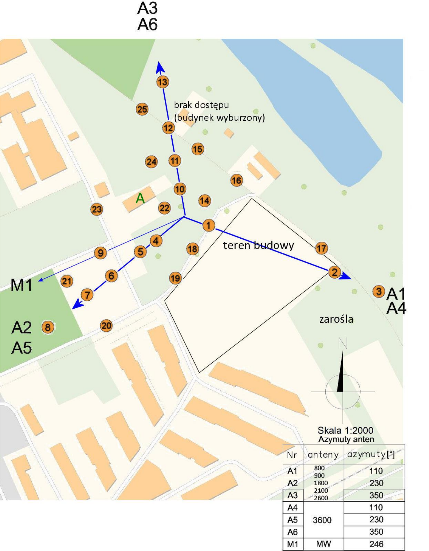
Zał. nr 2: Lokalizacja anten oraz ich azymuty, lokalizacja pionów (punktów) pomiarowych wokół instalacji radiokomunikacyjnej. -punkt (pion) pomiarowy.
