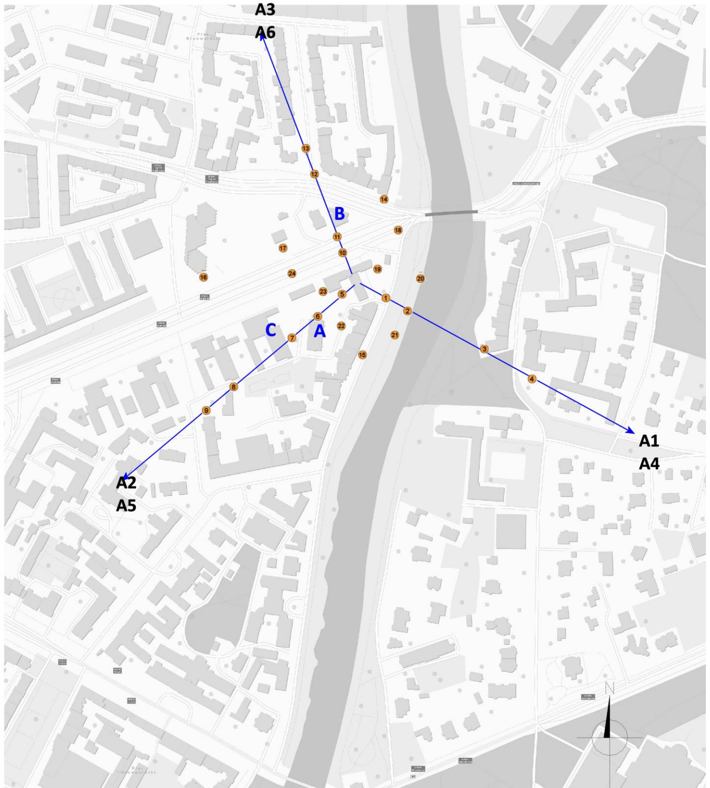
Azymuty anten
