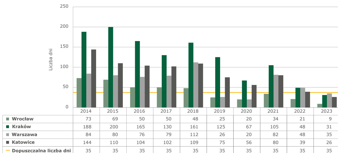
Wykres 60. Porównanie jakości powietrza we Wrocławiu, Krakowie, Warszawie, Katowicach w latach 2014–2023. Liczba dni z przekroczeniami dla pyłu zawieszonego PM 10 w poszczególnych miastach
