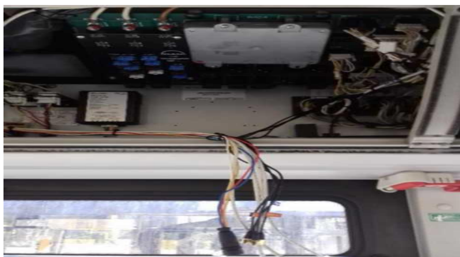
6.4. Wizualizacja montażu wsporników oraz połączeń elektrycznych instalacji OPS
