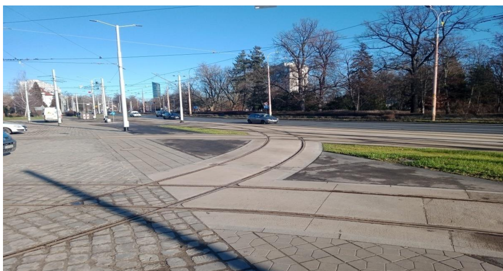
Fot. 72. Zmodernizowany węzeł rozjazdowy Zajeżdźni Borek
