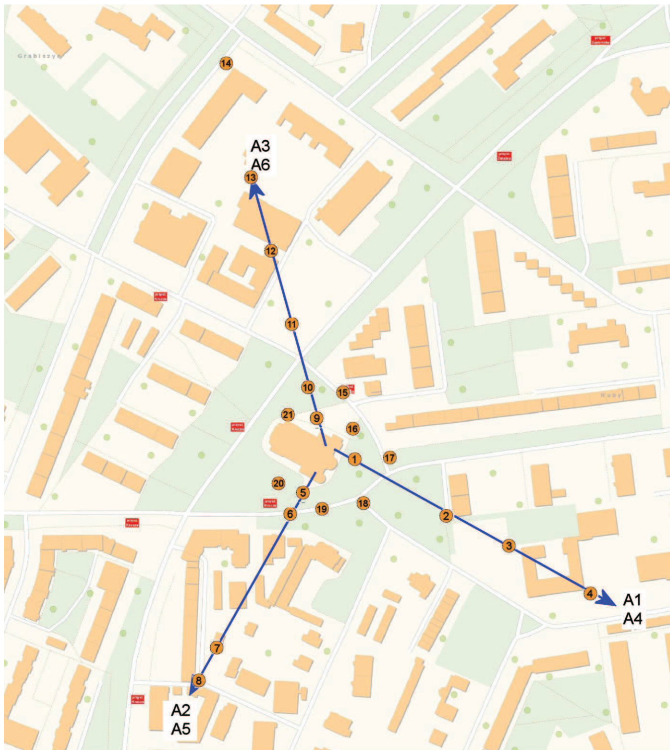
Azymuty anten
