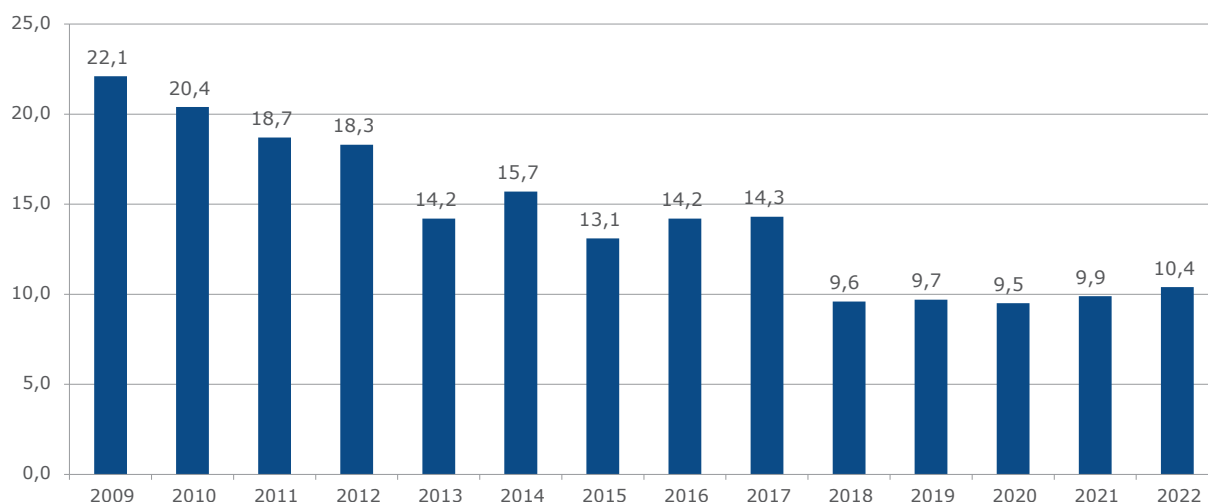
Wykres 63. Straty wody w sieci wodociągowej notowane przez MPWiK w latach 2009–2022 (w %)
