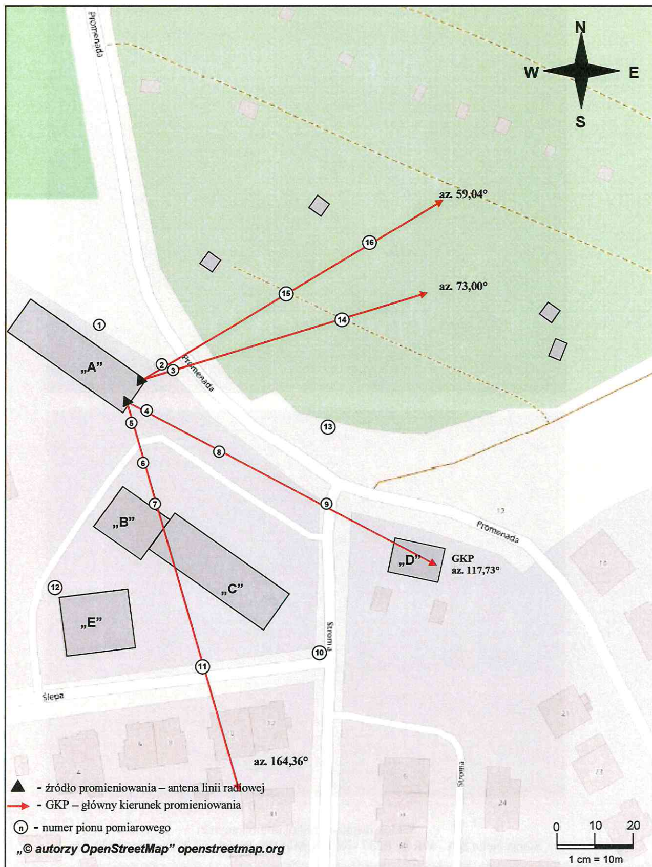
Rys. 1. Usytuowanie punktów i pionów pomiarowych w otoczeniu instalacji radiokomunikacyjnej Stacja Netia S.A. WROCB237-WROCM00190 Wrocław, ul. Promenada 11-13
