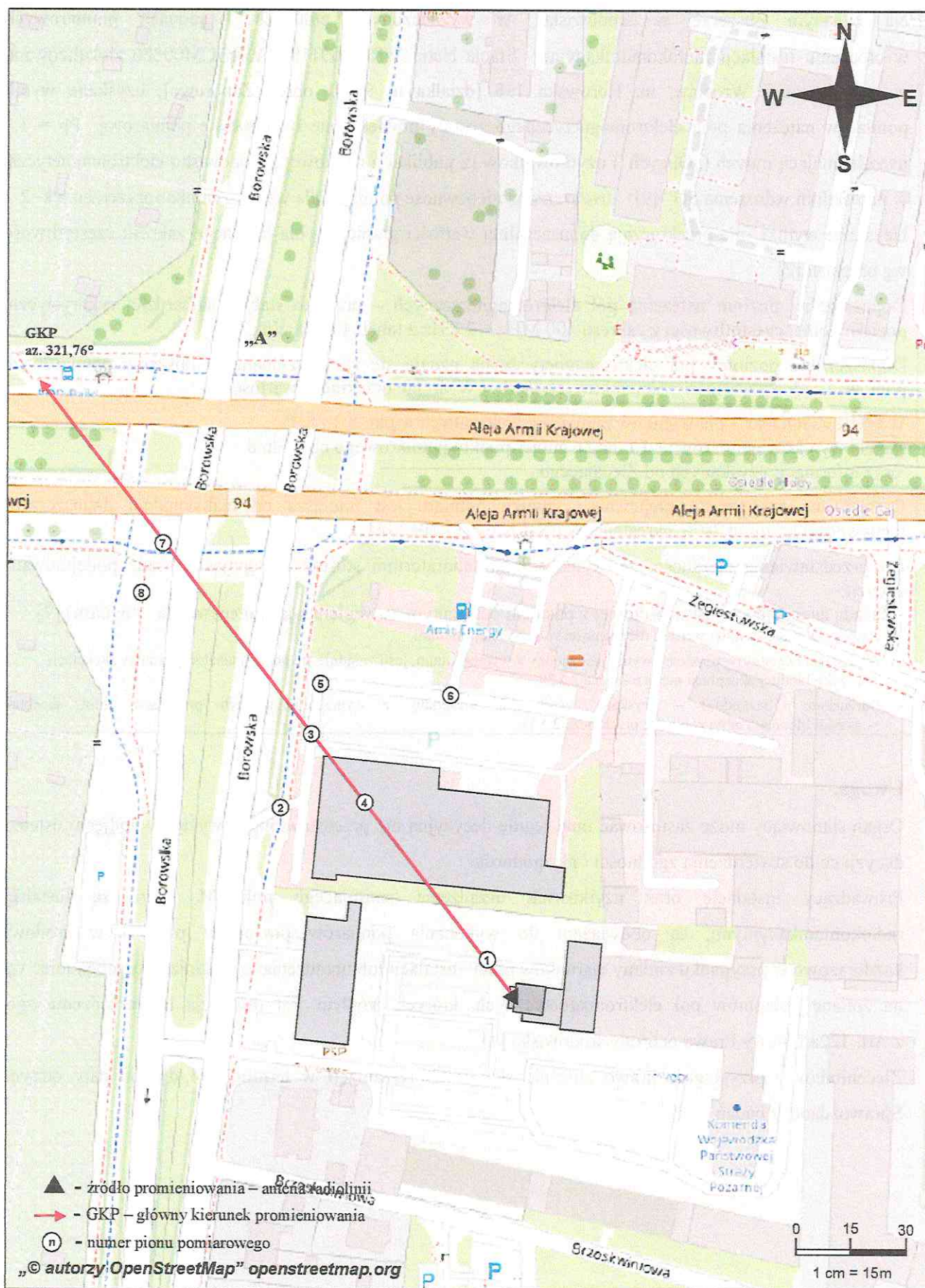
Rys. 1. Usytuowanie punktów i pionów pomiarowych w otoczeniu instalacji radiokomunikacyjnej Stacja Netia WROWD119-WROCM00886 Wrocław, ul. Borowska 138
