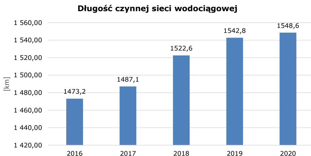
Rysunek 37. Długość eksploatowanej czynnej sieci wodociągowej (magistralnej i rozdzielczej) we Wrocławiu w latach 2016-2020 143
