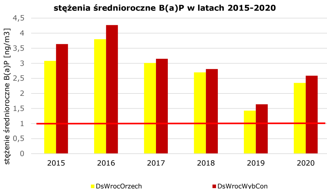
Rysunek 13. Przebieg stężenia średniorocznego benzo(a)pirenu w pył zawieszonym PM10 na poszczególnych stanowiskach pomiarowych w strefie aglomeracji wrocławskiej w latach 2015-2020 46
