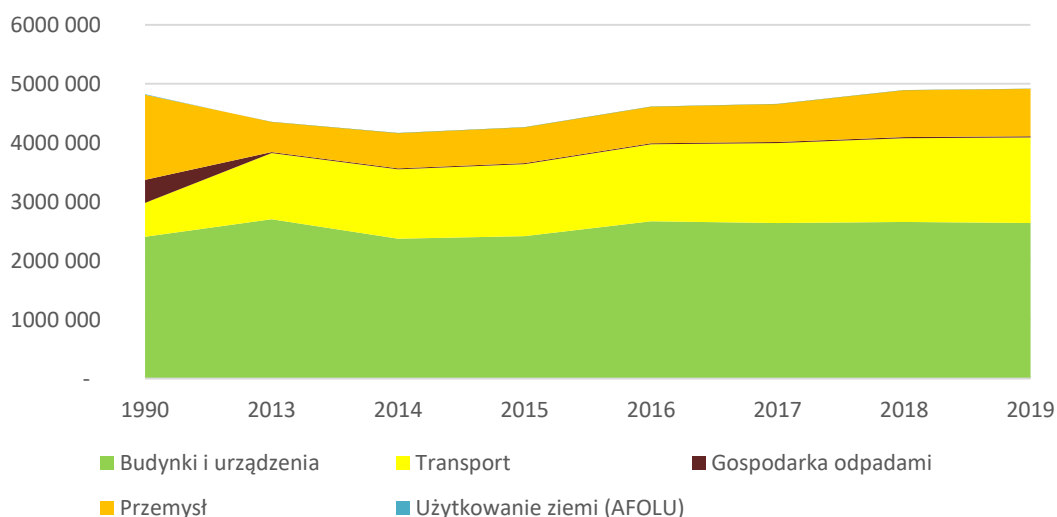
Rysunek 17. Zmiany wielkości emisji we Wrocławiu według sektorów w poszczególnych latach inwentaryzacji (okres 1990–2019) 56
