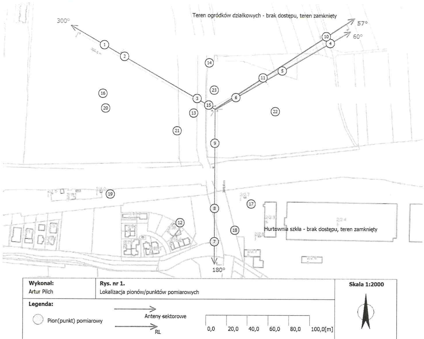
Rysunek 1 Lokalizacja pionów/punktów pomiarowych
